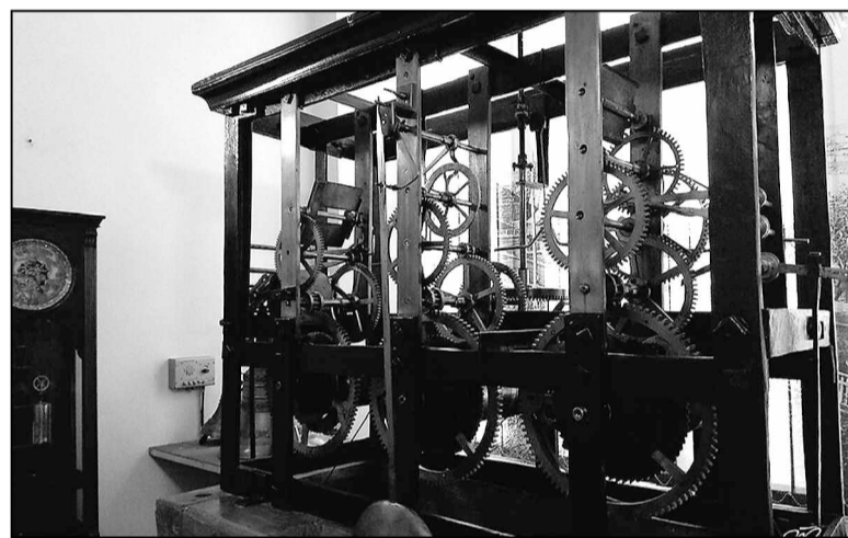
Механизм часов Алексея Трусова.
